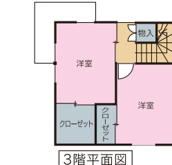
3階平面図
