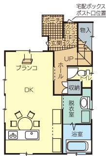
1階平面図
